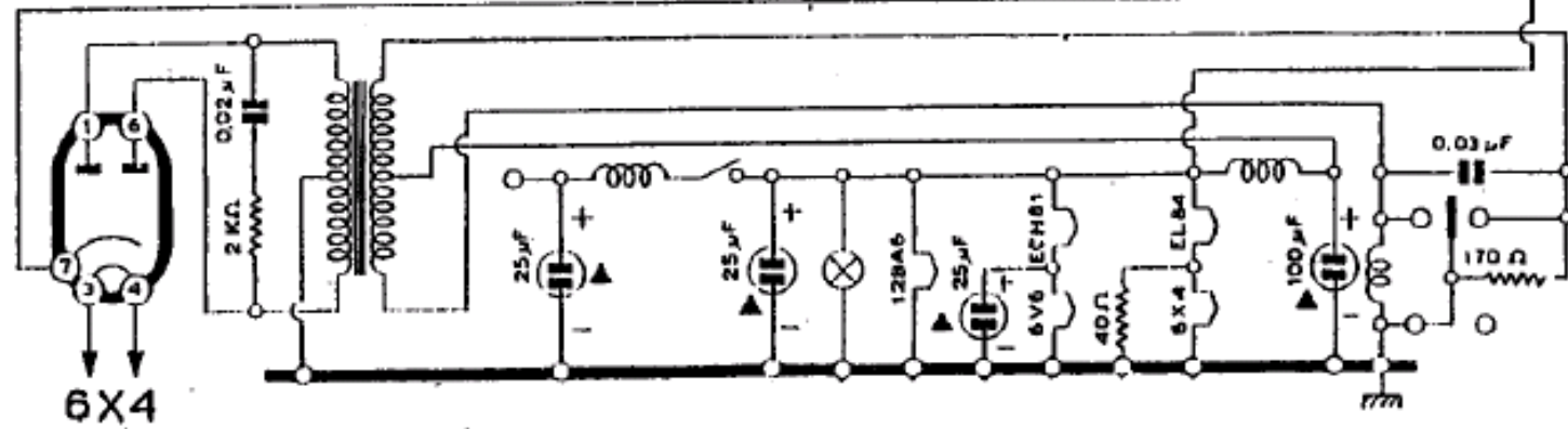
ASTER - Autoradio Modd. 513 - 563 - 613 - 663
